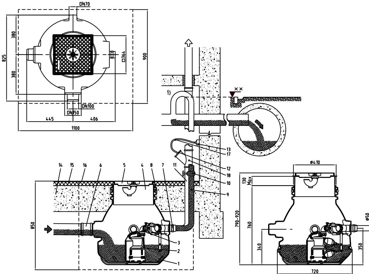
Abb. 2 Sanisett-Installationsbeispiel und Baumaße
