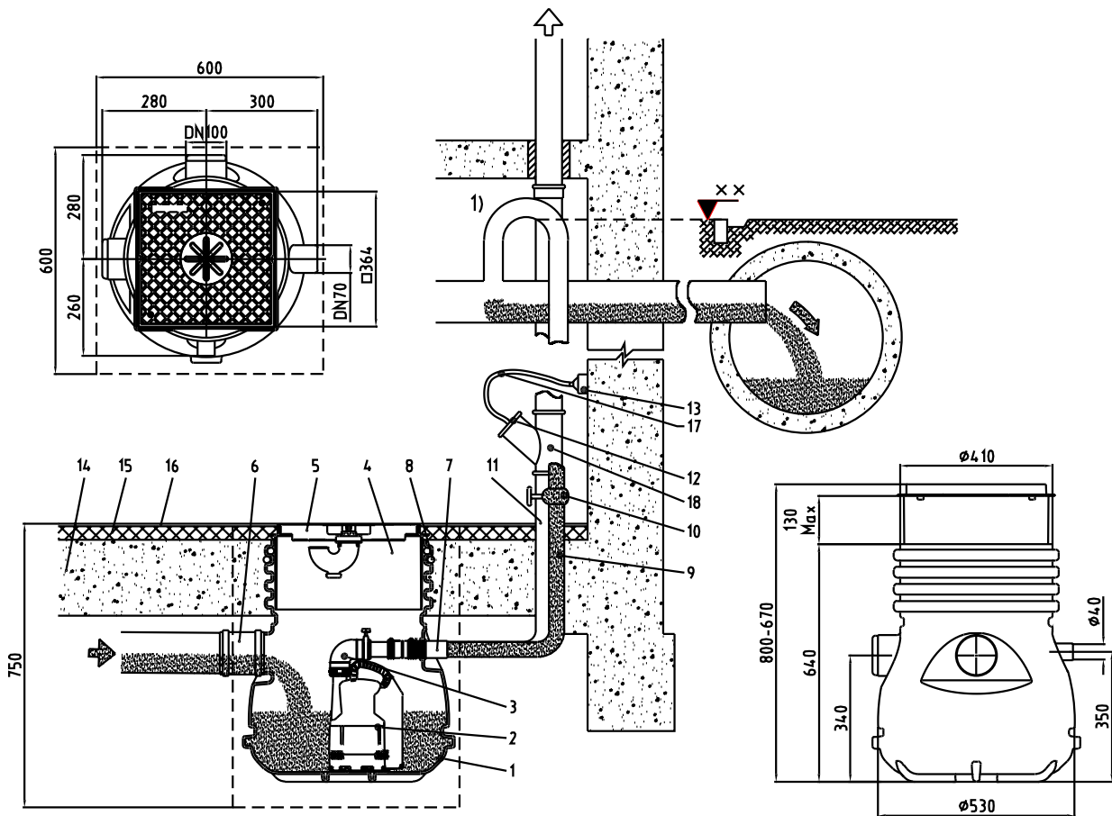
Abb. 1 Nirolift-Installationsbeispiel und Baumaße
