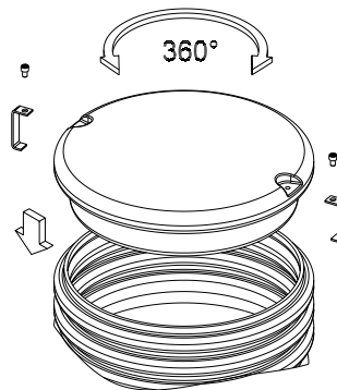
Abb. 6 Oberer Deckel des Sanisett
