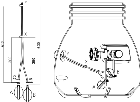
Abb. 4 Schwimmschaltereinbau bei Sanisett
